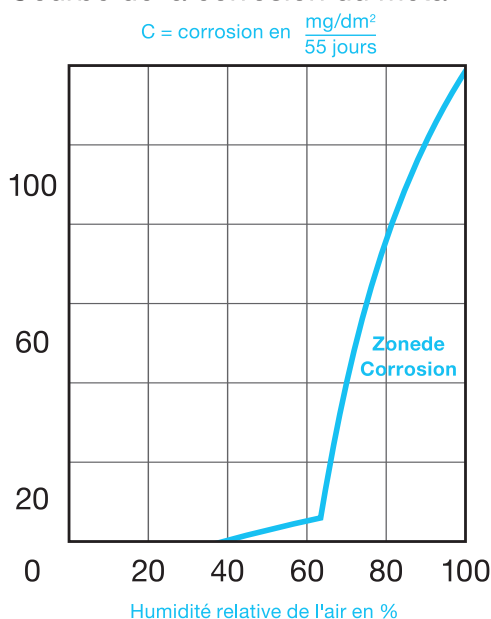
Courbe de la corrosion du métal.
